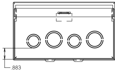
view A-A
