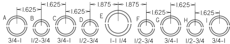
CONDUIT SIZES
