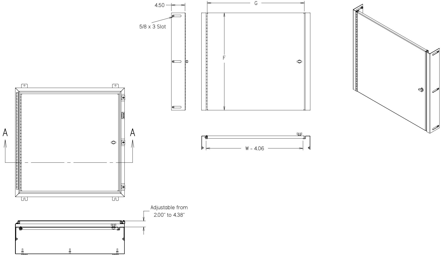
SECTION A-A
